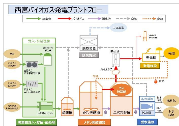
西宮バイオガス発電プラントフロー
